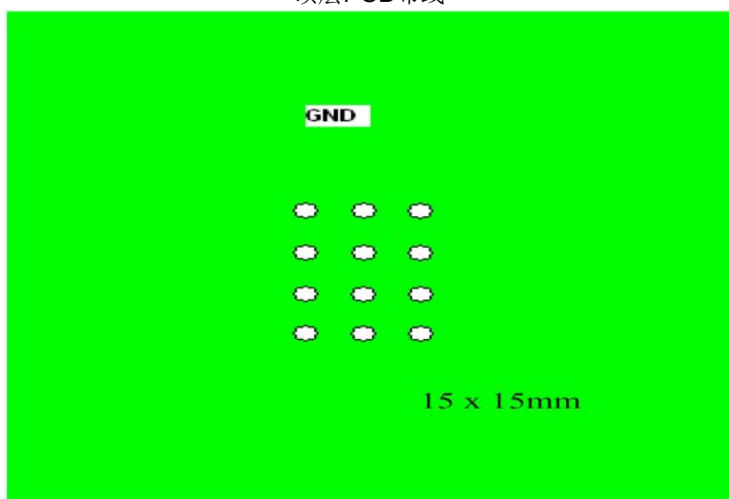
底层PCB布线
