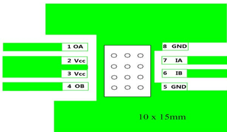
顶层PCB布线
