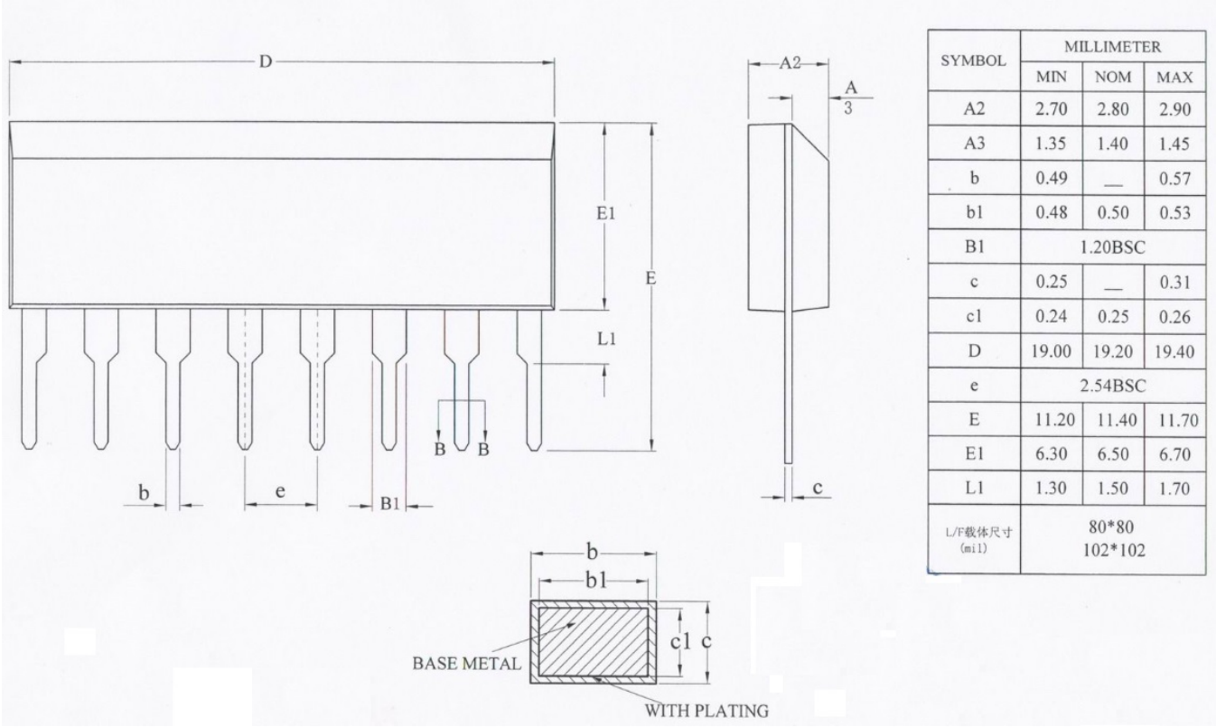
ESOP8封装
