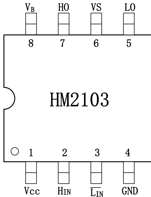
图 4-1. HM2103管脚定义
