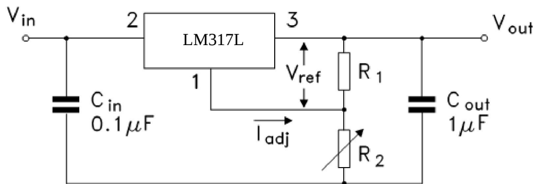
测试线路图
