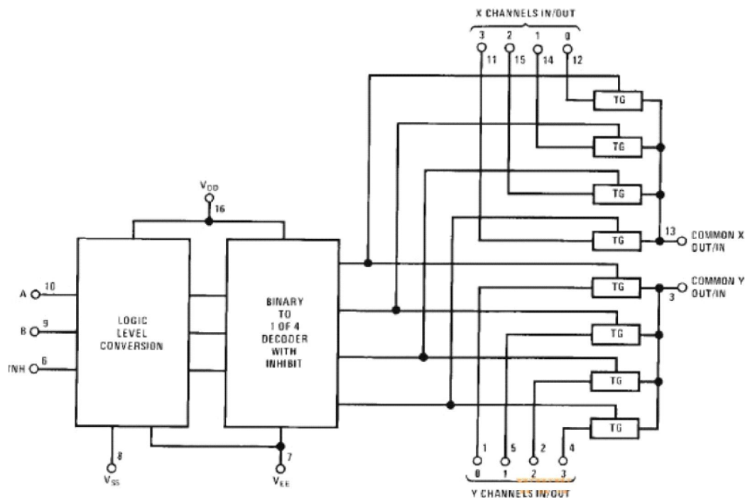
CD4052 逻辑图：
