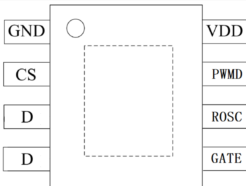
HM9808 图 2 管脚排列图
