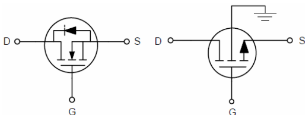
普通 MOSFET
