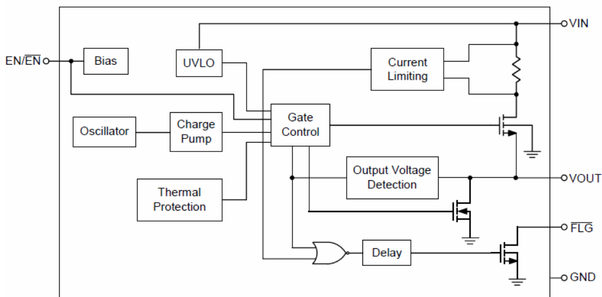
图 2 功能框图
