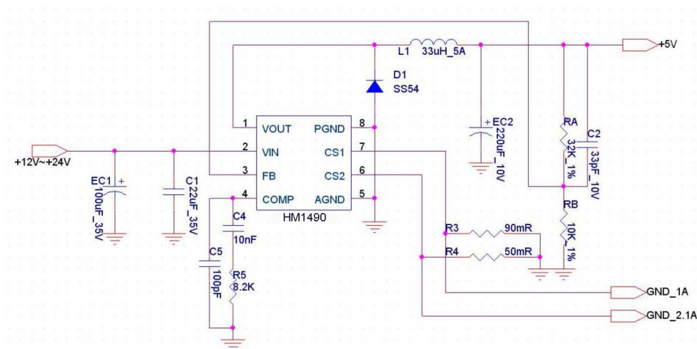
双路输出应用电路
