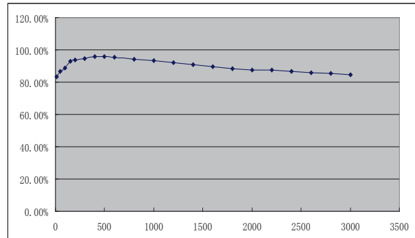
Vin=5V, Vout=3.3V
