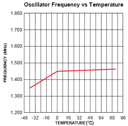
Vin=5V, Vout=3.3V
