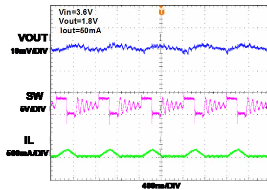
PFM MODE
