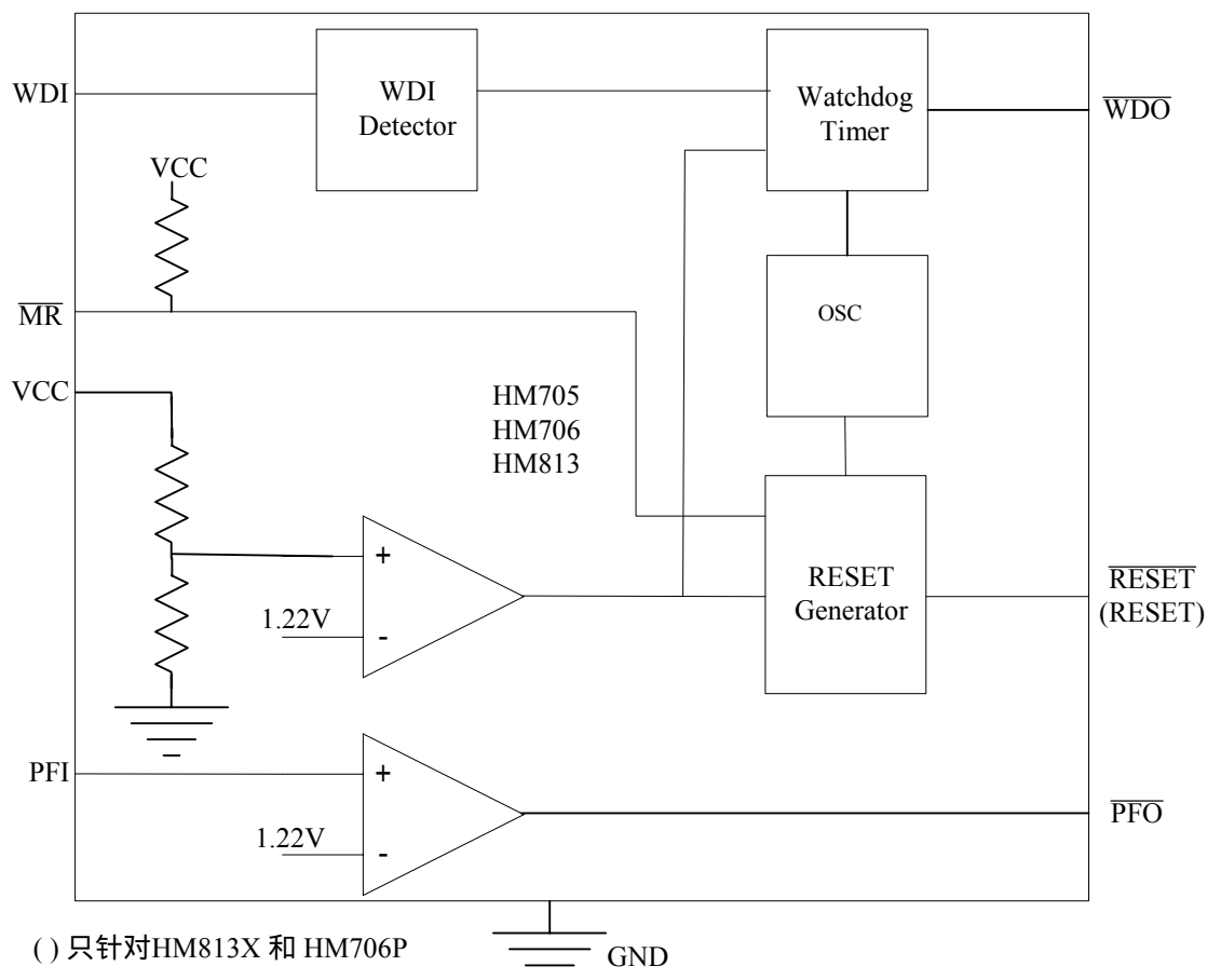
图 2 HM705/706X/813X 功能框图
