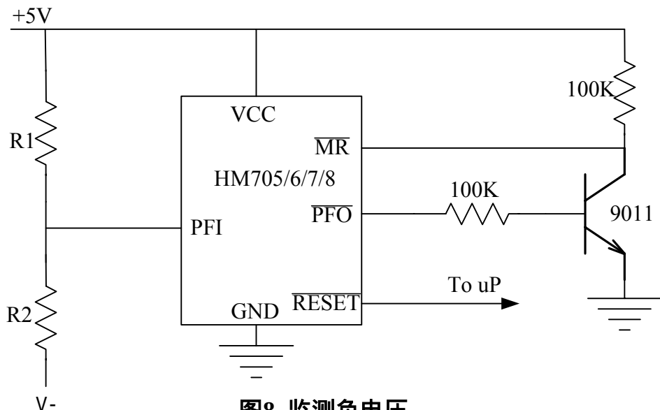
图8 监测负电压
