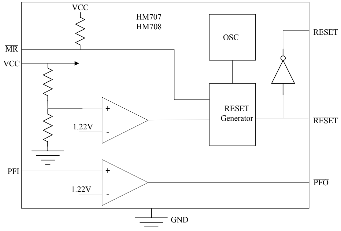
图 3 HM707/708X 功能框图
