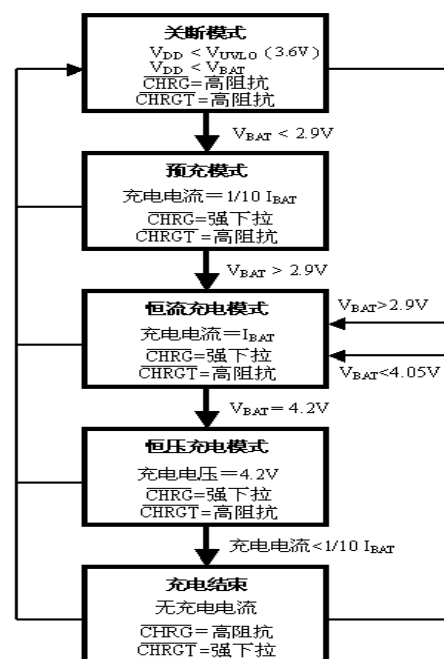
图1：一个典型充电循环的状态图
