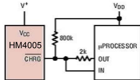
图 5：采用一个微处理器来确定引脚状态
