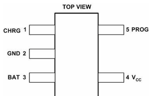
图 1. 封装
