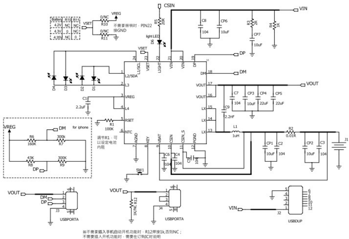
图 5 4LED 电量显示典型应用原理图
