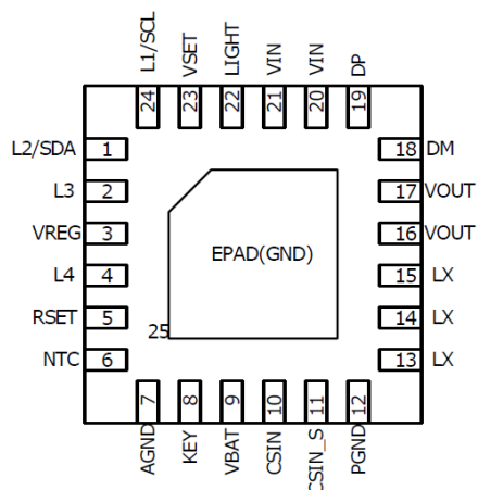
图 2 HM5919B 引脚图
