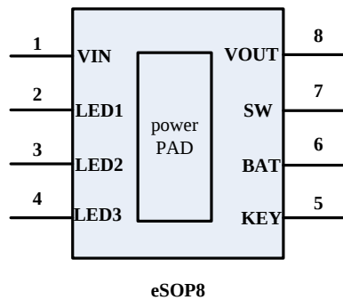
图 2 ( - 引脚图
