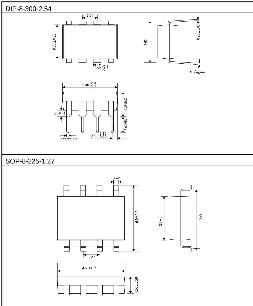
封装外形图
