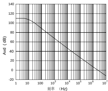
图 5 开环频率响应
