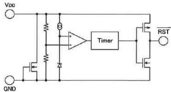
CMOS output
