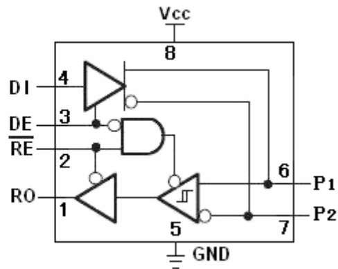
图 2: BL3085NE 逻辑图
